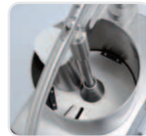
Particolare tramoggia guidata Guided feedbox detail
